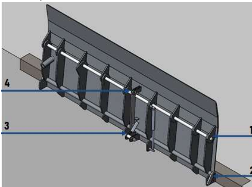
Рисунок 8 – Точки густой смазки
